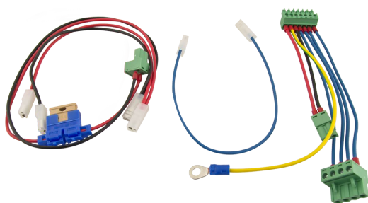
Zestaw wtyków i przewodów
